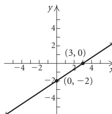
2x - 3y = 6
